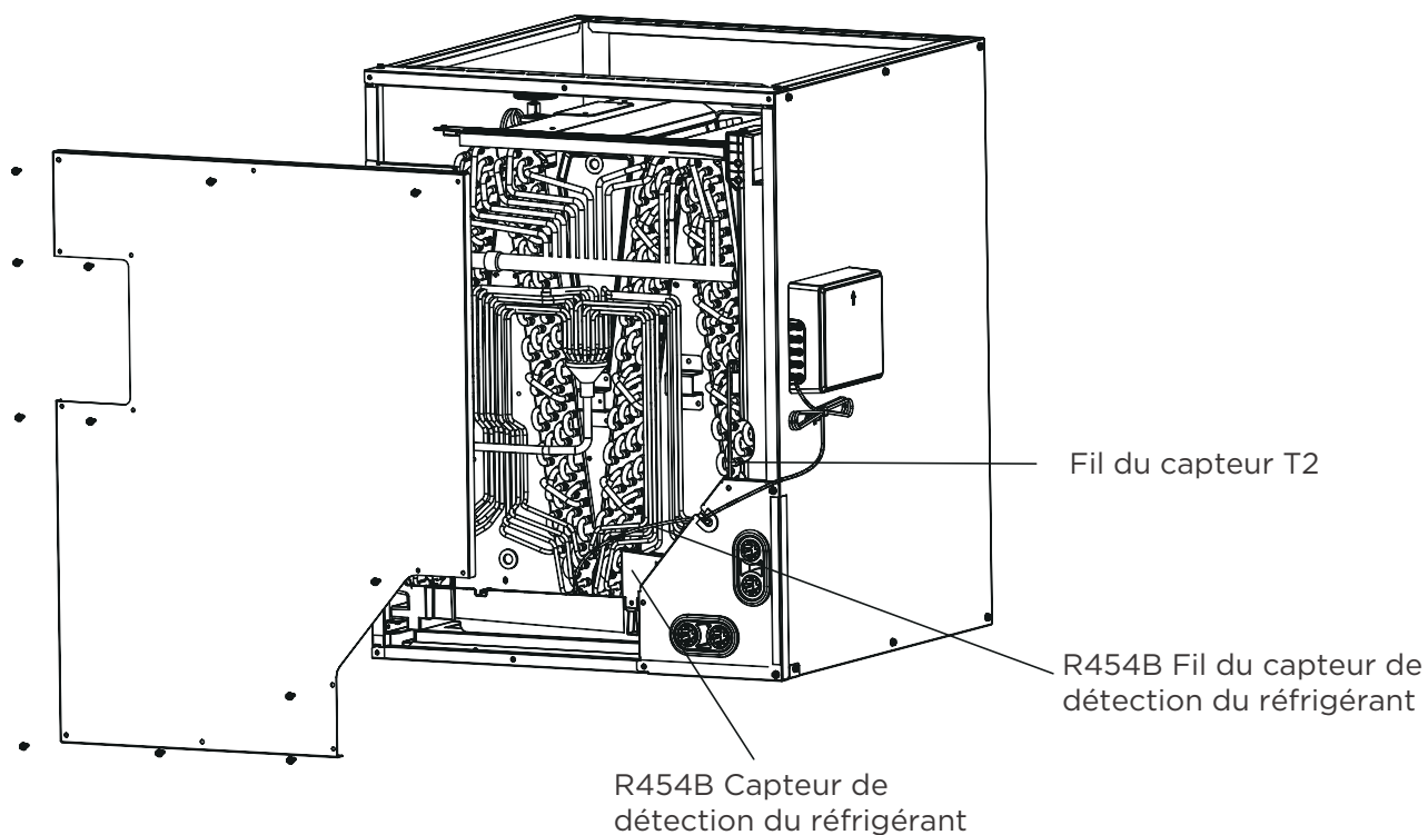
DIMENSIONS DU BOÎTIER ET EMPLACEMENT DES COMPOSANTS
