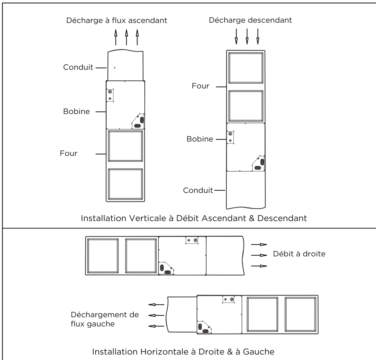
Type d'installation 2 : Modèle MVBM-60C28T6N10 installation de la bobine sur le four
