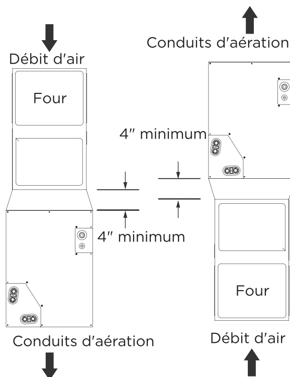
Installation verticale de débit ascendant et descendant
