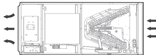
Horizontal left
