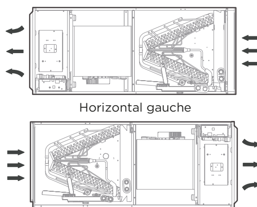
Horizontal droit
