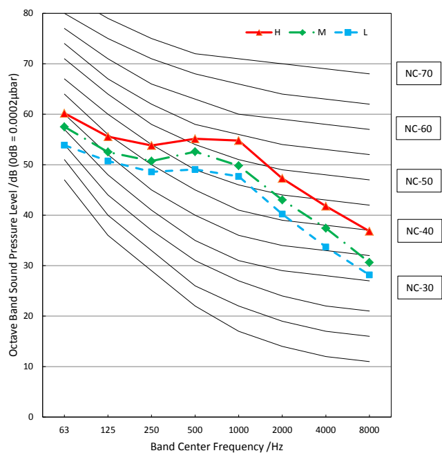
MTIU-18HWFN1-M
