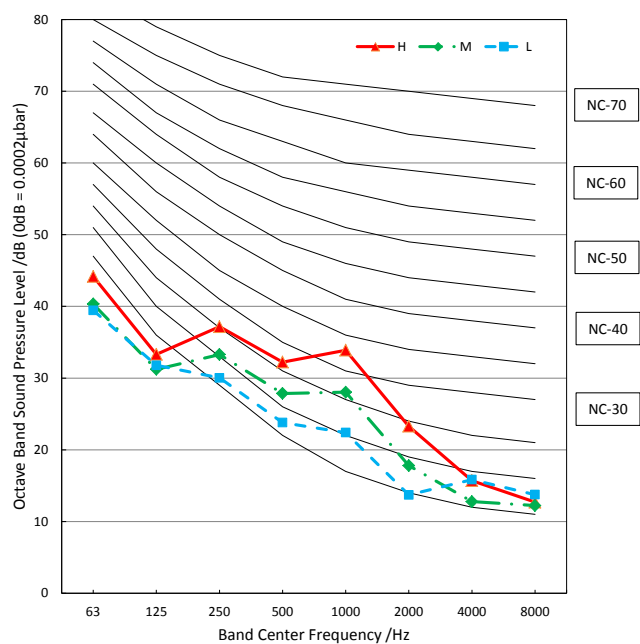
MTIU-18HWFN1-M
