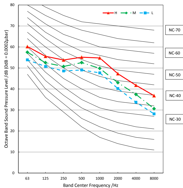
MTIU-24HWFN1-M
